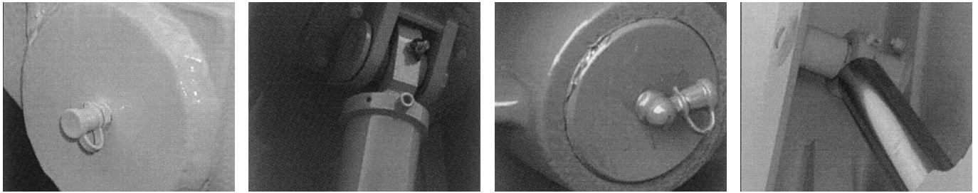
— Articulation de caisse — ————— Palier supérieur et inférieur du vérin ————— — Palier de vérin de porte —
